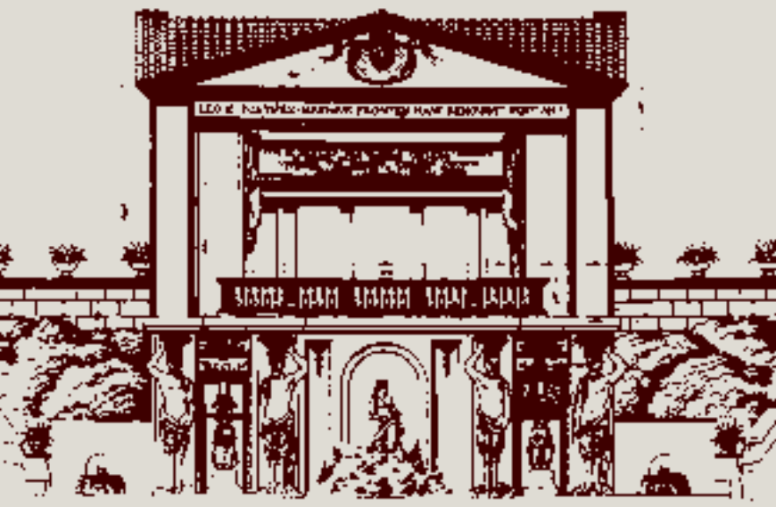
Fig. 42. Prospetto del Ninfeo, da Letarouilly, Le Vatican et la Basilique de Saint Pierre de Rome par Paul Letarouilly, Paris 1882, Fig. 6.
